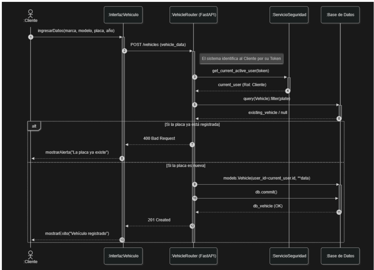
CU6- Gestionar Información del Vehículo
