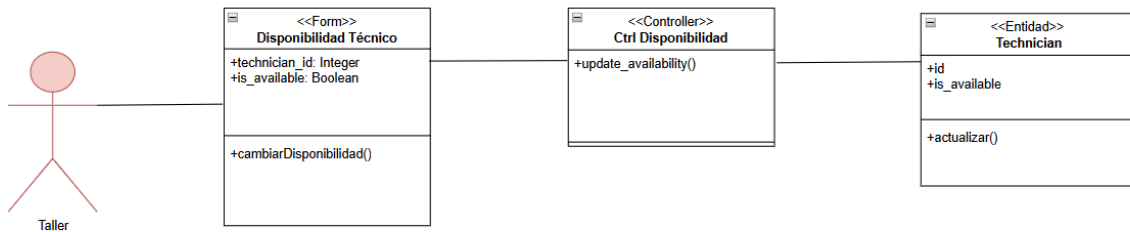
CU12-Gestionar Disponibilidad de Técnicos
