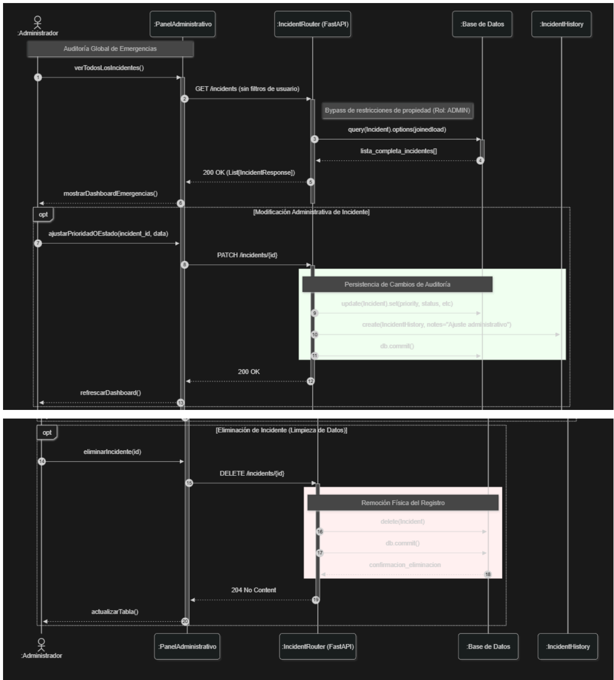
CU20. Bitácora del Sistema
