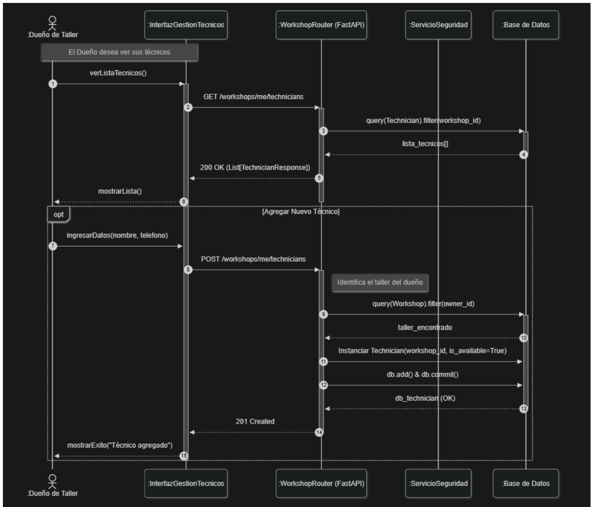
CU12. Gestionar disponibilidad de técnicos
