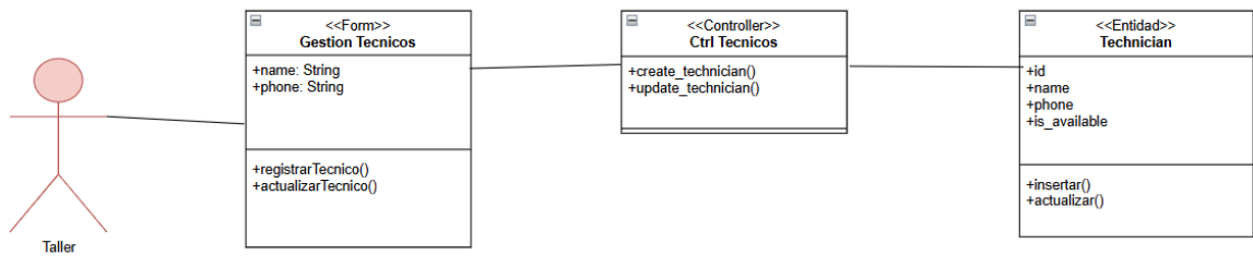
CU11 - Gestionar Técnicos del Taller
