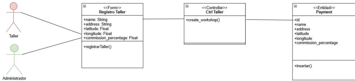
CU10 - Registrar Taller
